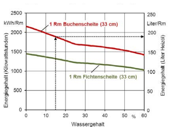
Der Wassergehalt beeinflusst den Energiegehalt eines Holzstapels (Unterhalb von 25 % Wassergehalt beginnt die Schrumpfung)
